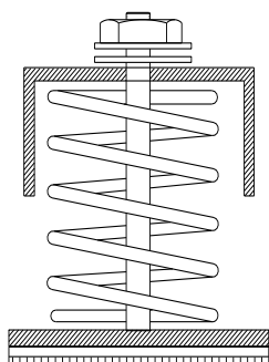
(1) 阻尼钢弹簧减振器
