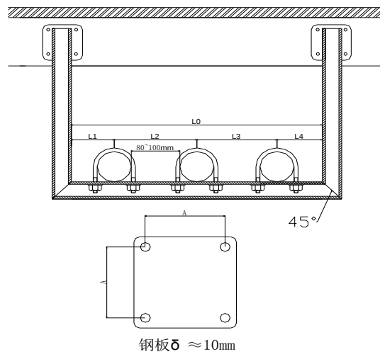
(2) 槽钢支架制作方法
