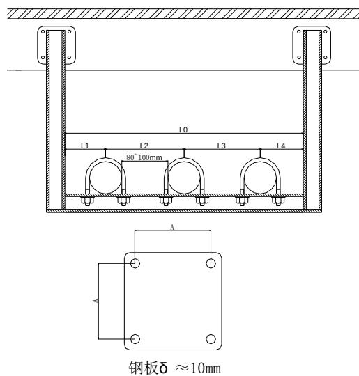
(4) 槽钢支架制作方法
